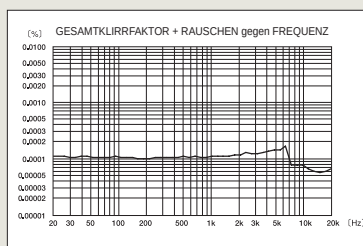
Gesamtklirrfaktor (einschl. Rauschen) gegen Frequenzgang
