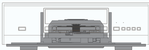
Das SA-CD/CD-Laufwerk liegt niedrig im Gerät, um diesem einen niedrigen Schwerpunkt zu verleihen
