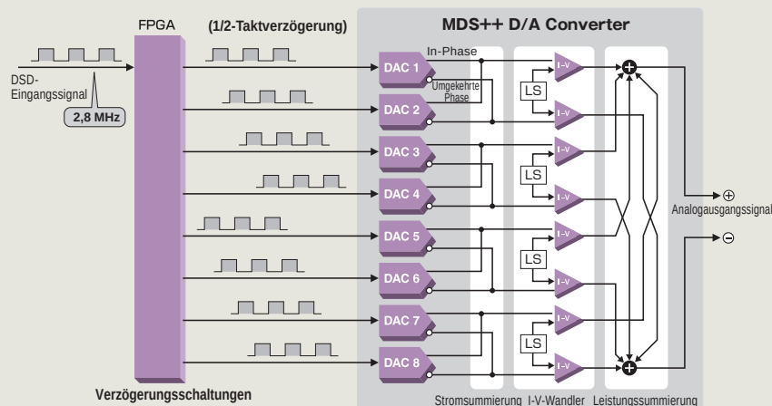
Blockschaltbild des MDSD-Prinzips
