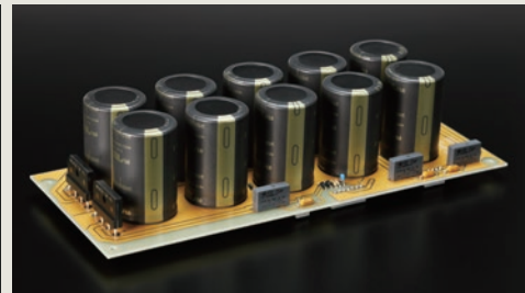
Rauscharme Stromversorgungskreise mit zehn Siebkondensatoren à 4.700 µF
