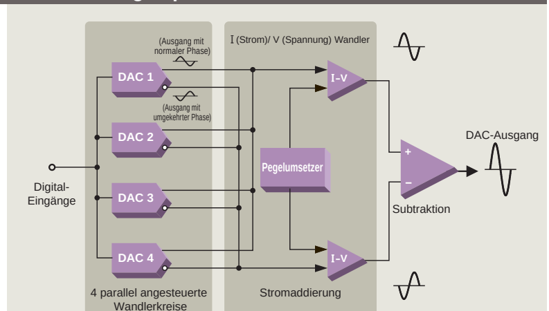
■ Blockdiagramm des D/A-Wandlers vom 4MDS+-Typ
