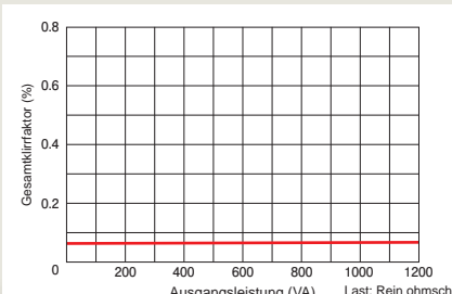
Ausgangsleistung – Gesamtklirrfaktor
