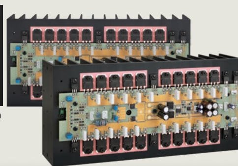
Ausgangsstufe mit zwanzigfach paralleler Gegenaktanordnung
