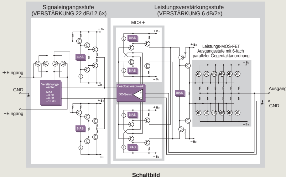
Schaltbild
