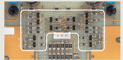
2-fach parallele Schaltungsanordnung der MCS+-Architektur
