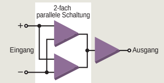
MCS+-Schaltungsarchitektur
