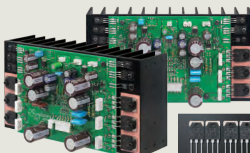
Leistungsverstärker
