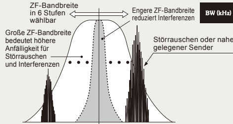
ZF-Filter mit variabler Bandbreite
