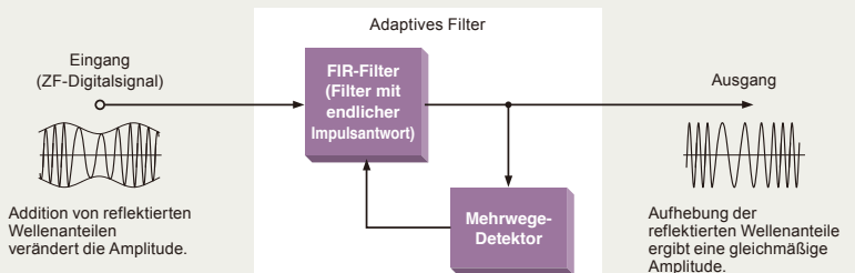
Funktion zur Unterdrückung von Mehrwegeempfang
